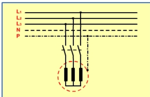
b. Gambar pengawatan saklar kutub tiga
