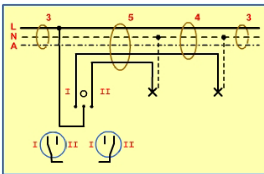
b. Gambar pengawatan listrik saklar kelompok
