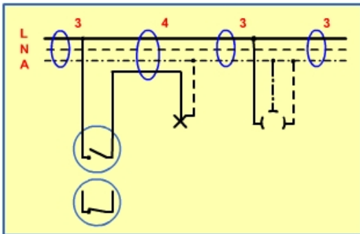
b. Gambar pengawatan saklar kutub tunggal
