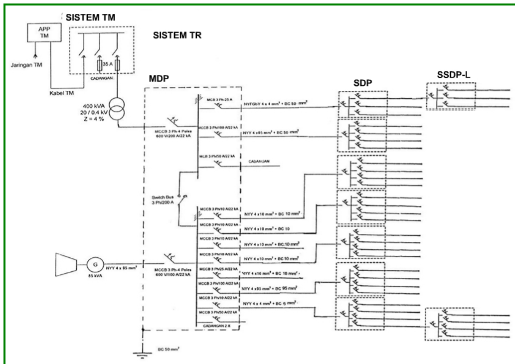
Gambar 2.12 Diagram satu garis instalasi listrik pada bangunan / gedung sistem Tegangan Menengah dan Tegangan Rendah
