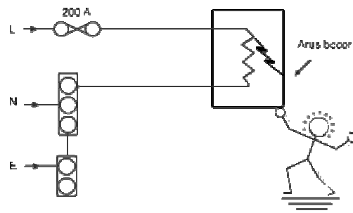
Gambar 1.11 Kondisi tegangan sentuh pada mesin
