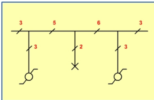
c. Gambar saluran saklar tukar
