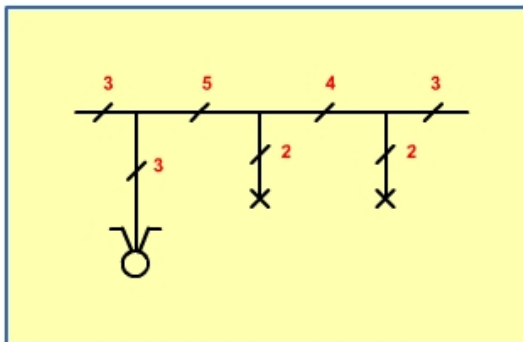
c. Gambar saluran saklar seri
