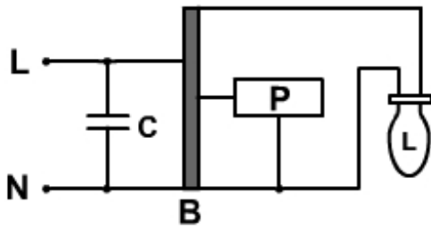
Gambar 2.87 Rangkaian dasar lampu sodium tekanan tinggi
