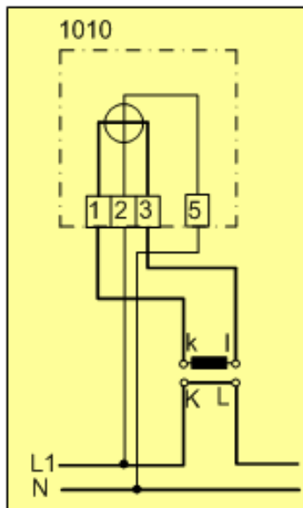
Gambar 2.17 Rangkaian Kwh satu fasa dengan trafo arus
