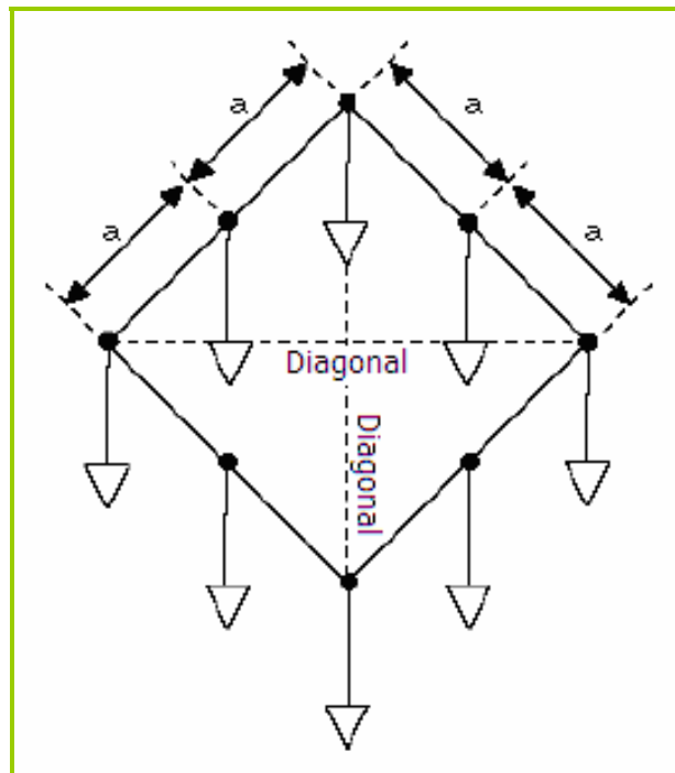
Gambar 2.123 Sistem Multi-elektroda
