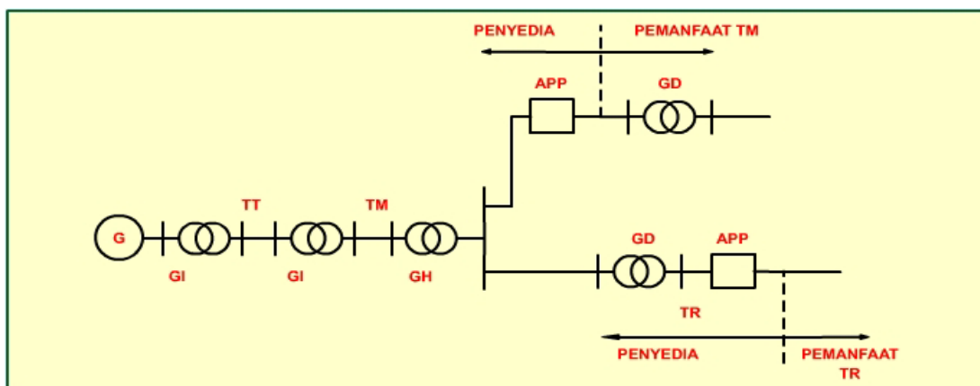
Gambar 2.5 Instalasi Penyediaan dan Pemanfaatan Tenaga Listrik
