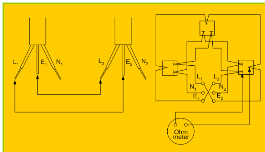
Gambar 2.135 Pengukuran resistansi kawat penghantar melingkar fasa dan pembumian
