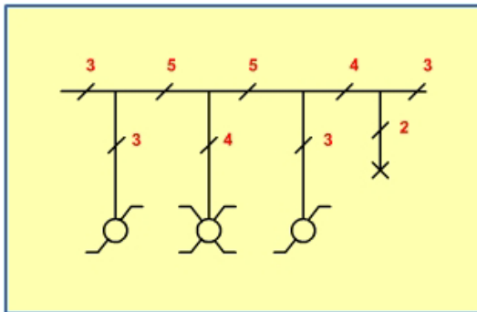
c. Gambar saluran saklar silang
