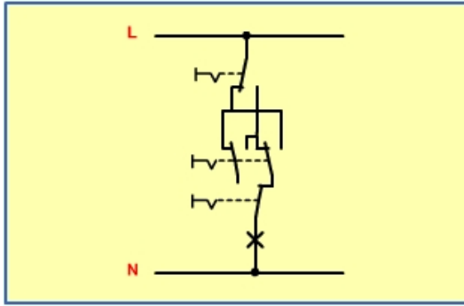
a. Gambar rangkaian listrik saklar silang
