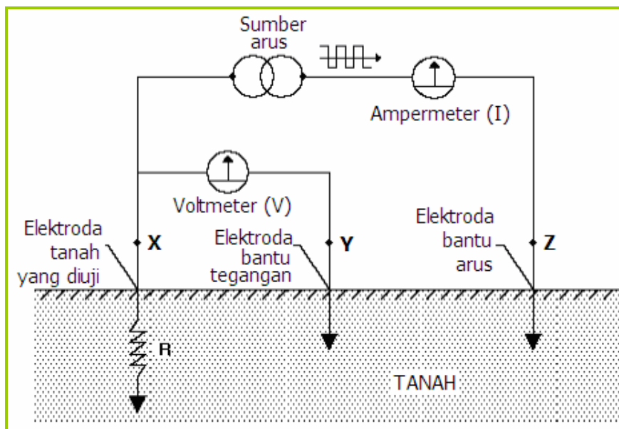
Gambar 2.117 Prinsip pengukuran tahanan elektroda pentanahan menggunakan metoda jatuh tegangan – 3 titik
