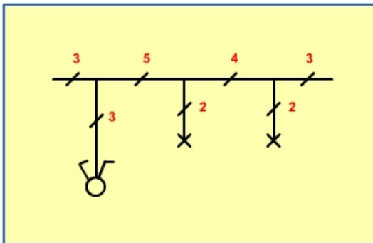
c. Gambar saluran listrik saklar kelompok
