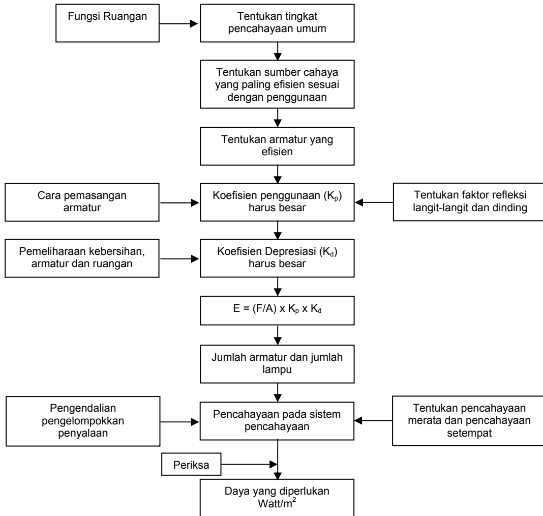
Gambar 2.56 Prosedur perencanaan teknis pencahayaan buatan
