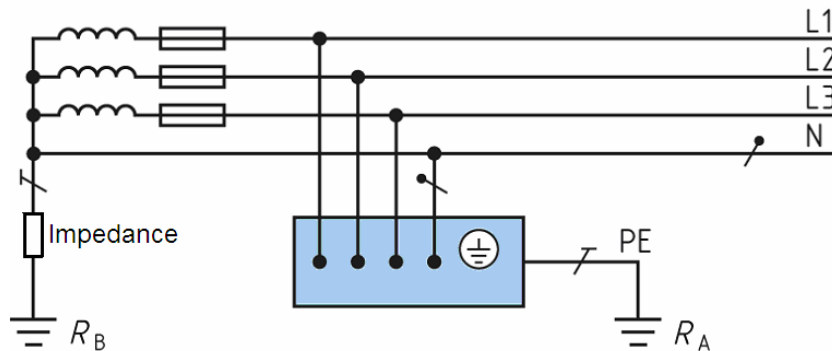
Gambar 2.109 Saluran Tanah Melalui Impedansi (IT)
