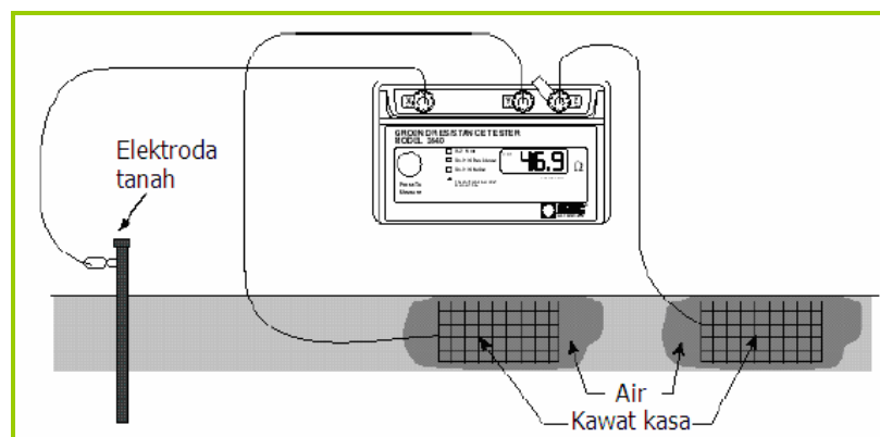
Gambar 2.131 Penggunaan kawat kasa sebagai pengganti dari elektroda bantu
