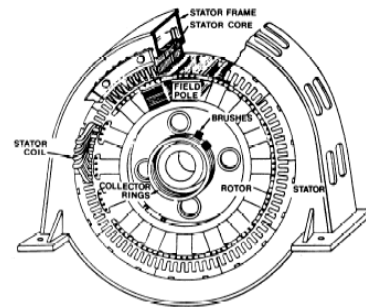
c. Generator secara umum
