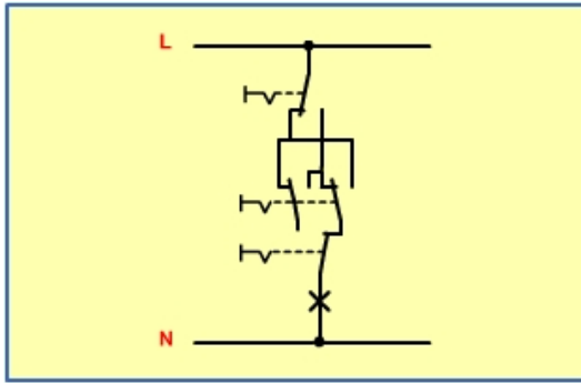
a. Gambar rangkaian listrik saklar tukar
