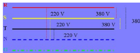
(b) Fasa-Tiga
