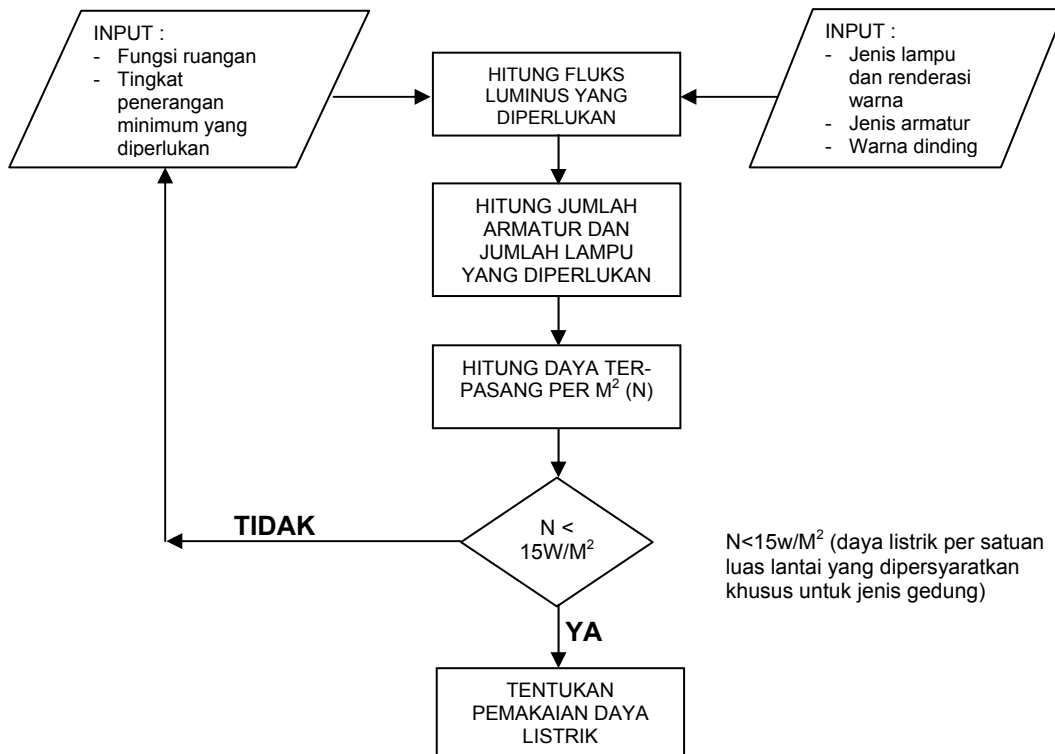
Gambar 2.55 Diagram perhitungan dan optimasi daya listrik pada sistem pencahayaan buatan
