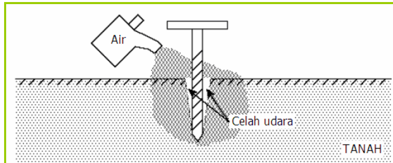
Gambar 2.130 Cara mengatasi tahanan kontak antara elektroda dengan tanah sekitarnya
