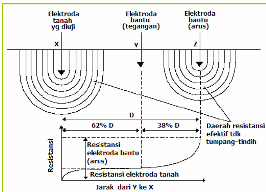
Gambar 2.122 Daerah pengukuran 62%
