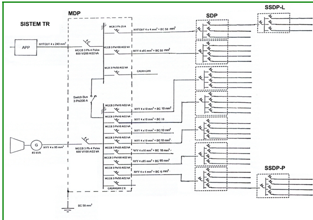
Gambar 2.11 Diagram satu garis instalasi listrik pada bangunan / gedung Tegangan Rendah
