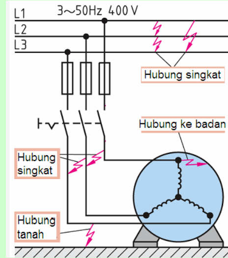
Gambar 1.30 Jenis Arus Kesalahan
