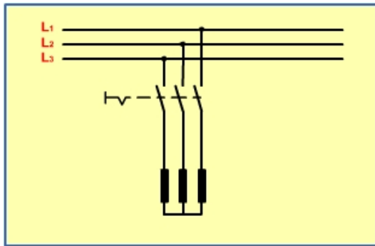
a. Gambar rangkaian listrik saklar kutub tiga
