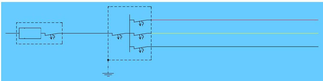
Gambar 2.36 Diagram satu garis
