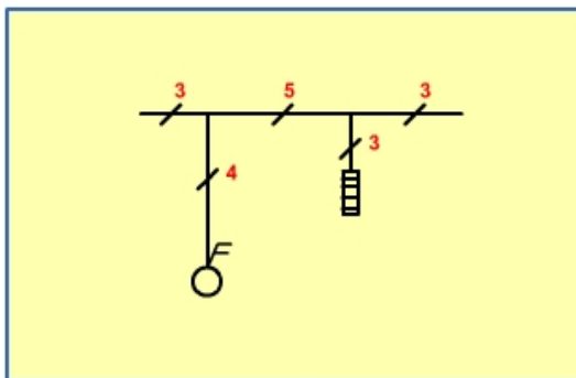
c. Gambar saluran saklar kutub ganda
