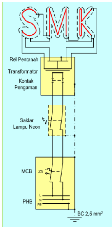
Gambar 2.78 Contoh Lampu Reklame
