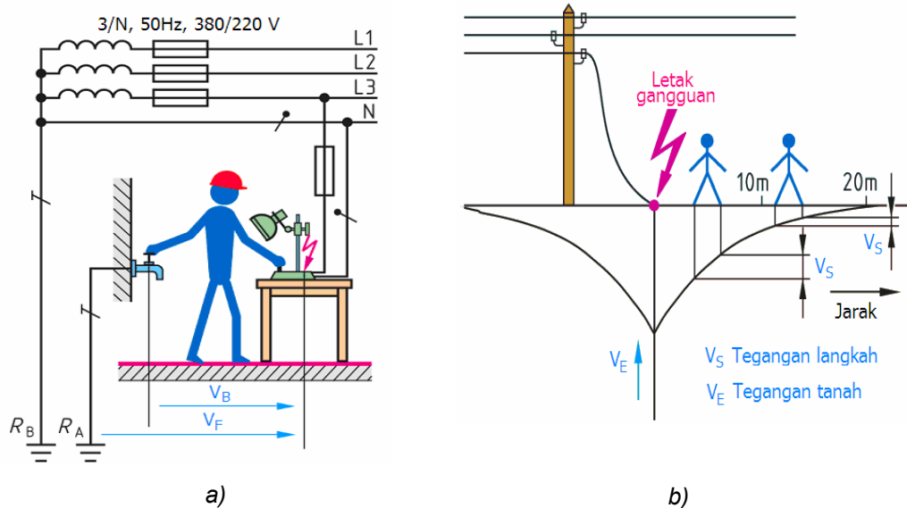
Gambar 2.111 Tegangan sentuh dan tegangan langkah
