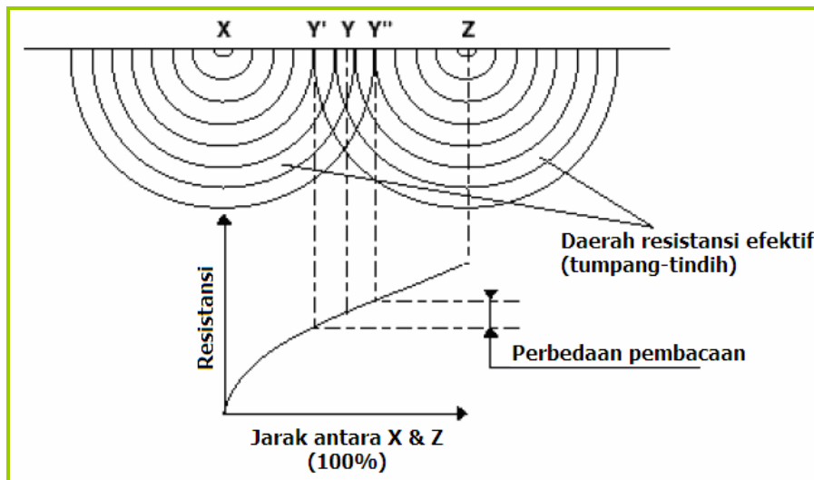
Gambar 2.118 Daerah resistansi efektif dari dua elektroda yang tumpang-tindih
