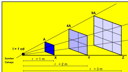
Gambar 2.49 Hukum kebalikan kuadrat iluminasi
