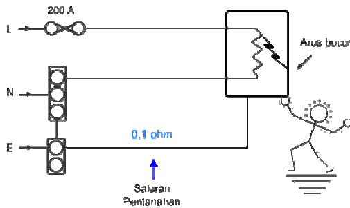
Gambar 1.12 Saluran pentanahan sebagai pengaman terhadap tegangan sentuh
