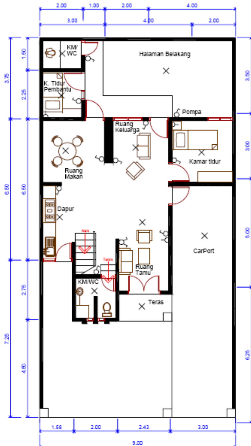
Gambar 2.9 Denah rumah tipe T-125 lantai dasar
