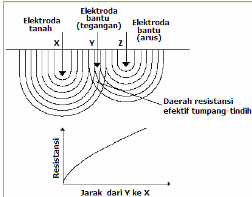
Gambar 2.121 Daerah resistansi efektif tumpang-tindih
