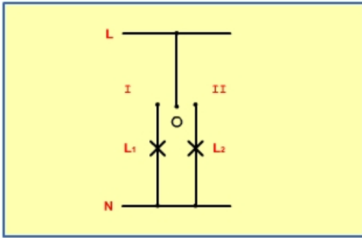
a. Gambar rangkaian listrik saklar kelompok
