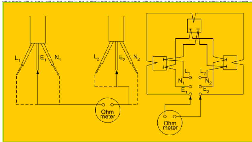
Gambar 2.133 Pengukuran resistansi kawat fasa, netral dan pembumian
