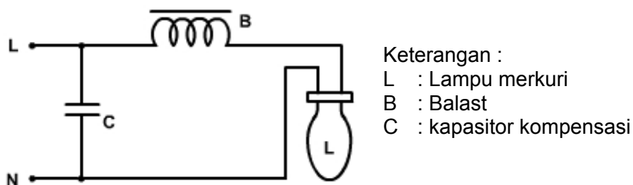
Gambar 2.80 Rangkaian dasar lampu merkuri tekanan tinggi
