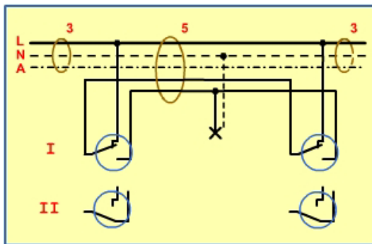
b. Gambar pengawatannya
