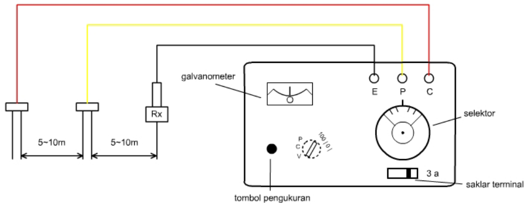
Gambar 2.115 Pengukuran Metoda 3 Kutub
