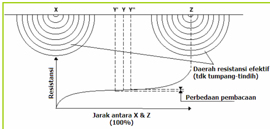
Gambar 2.119 Posisi elektroda Y di luar daerah resistansi efektif dari dua elektroda yang tidak tumpang-tindih
