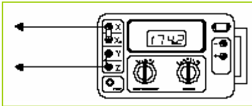
Gambar 2.125 Pengukuran kontinuitas hantaran pentanahan
