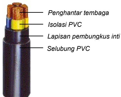
Gambar 2.29 Kabel NYY
