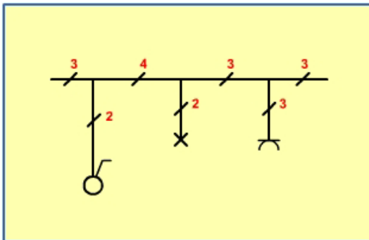
c. Gambar saluran saklar kutub tunggal
