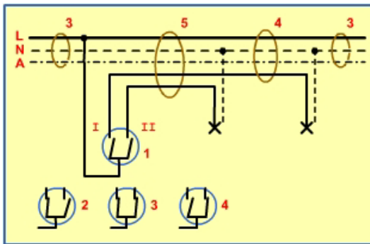
b. Gambar pengawatan saklar seri
