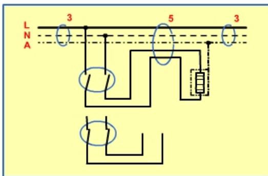
b. Gambar pengawatan saklar kutub ganda
