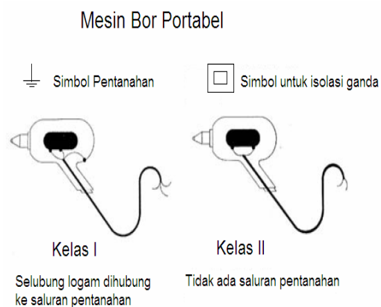
Gambar 1.16. Contoh klasifikasi pengamanan alat portabel
