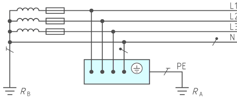
Gambar 2.108 Saluran Tanah Sistem dan Saluran Bagian Sistem Terpisah (TT)
