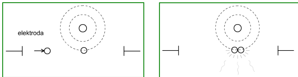
Gambar 2.76 Gerakan elektron gas
