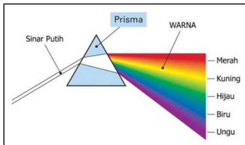
Gambar 2.39 Warna-warna Spektrum
