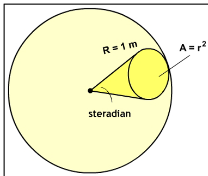
Gambar 2.45 Steradian
