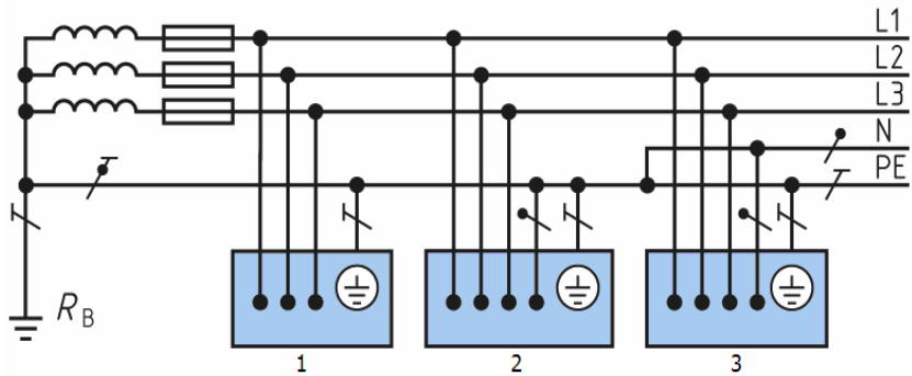
Gambar 2.106 Saluran Tanah dan Netral disatukan pada sebagian sistem (TN-C-S)
