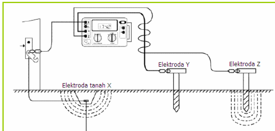
Gambar 2.127 Cara menetralkan noise dengan melilitkan kabel-kabel ukur secara bersama-sama
