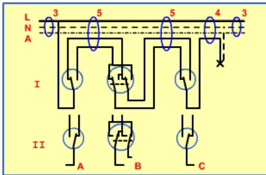
b. Gambar pengawatan saklar silang
