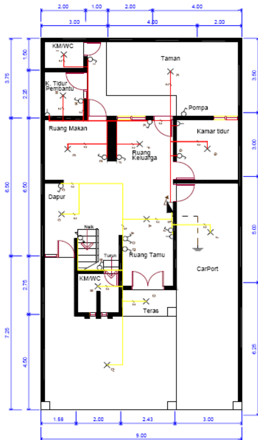
Gambar 2.10 Instalasi rumah tipe T-125 lantai dasar
