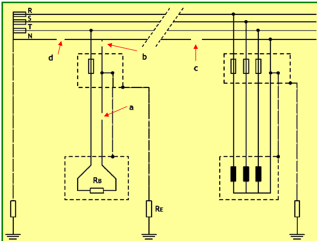
Gambar 2.132 Kasus putusnya penghantar netral pada sistem PNP
