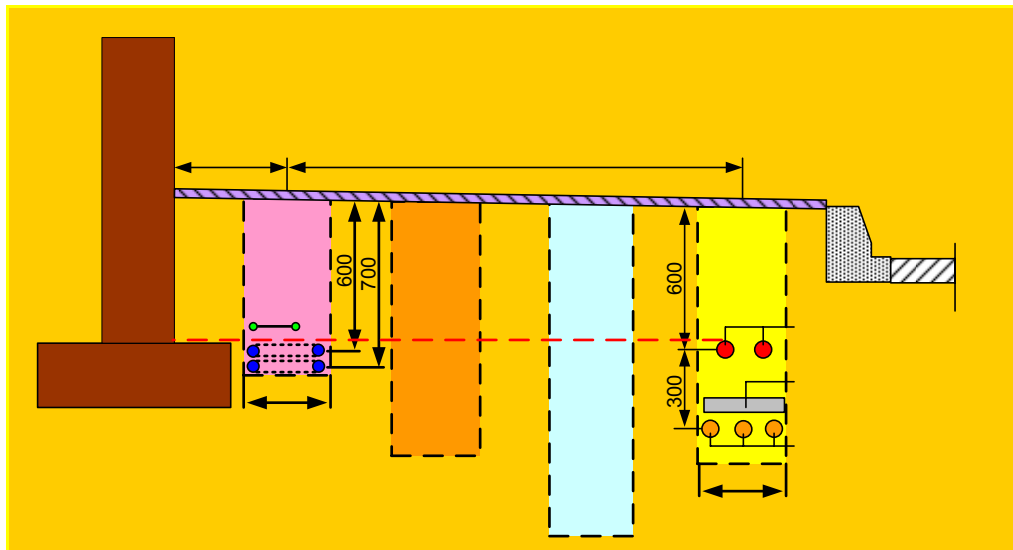
Gambar 2.37 Saluran instalasi bawah trotoar
