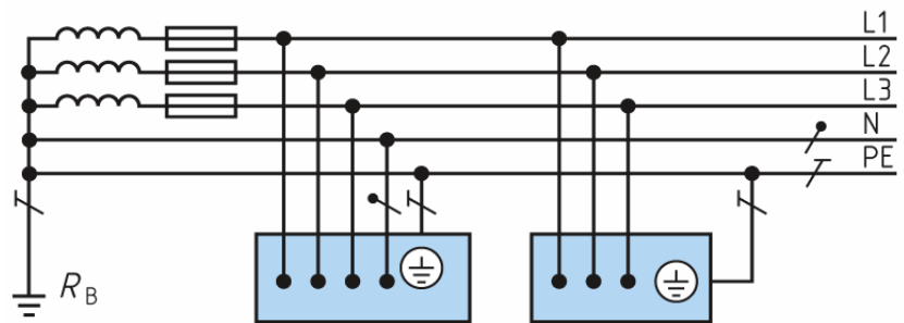
Gambar 2.107 Saluran Tanah dan Netral dipisah (TN-S)
