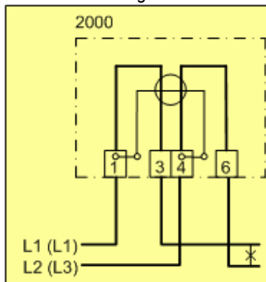
Gambar 2.18 Rangkaian Kwh dua fasa dengan sambungan tetap
