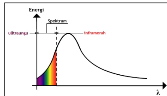
Gambar 2.40 Energi – Panjang Gelombang – Lampu Pijar 500W
