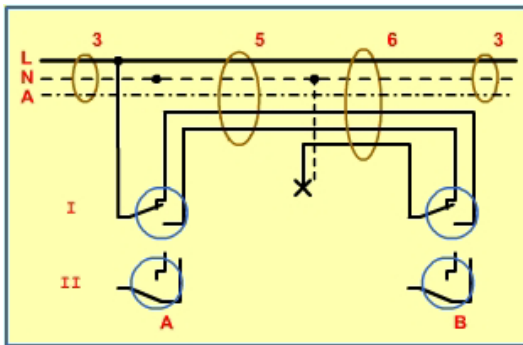
b. Gambar pengawatan saklar tukar
