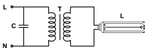
Gambar 2.85 Rangkaian dasar lampu sodium tekanan rendah
