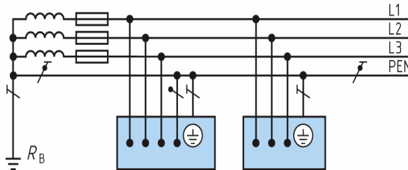
Gambar 2.105 Saluran Tanah dan Netral disatukan (TN-C)
