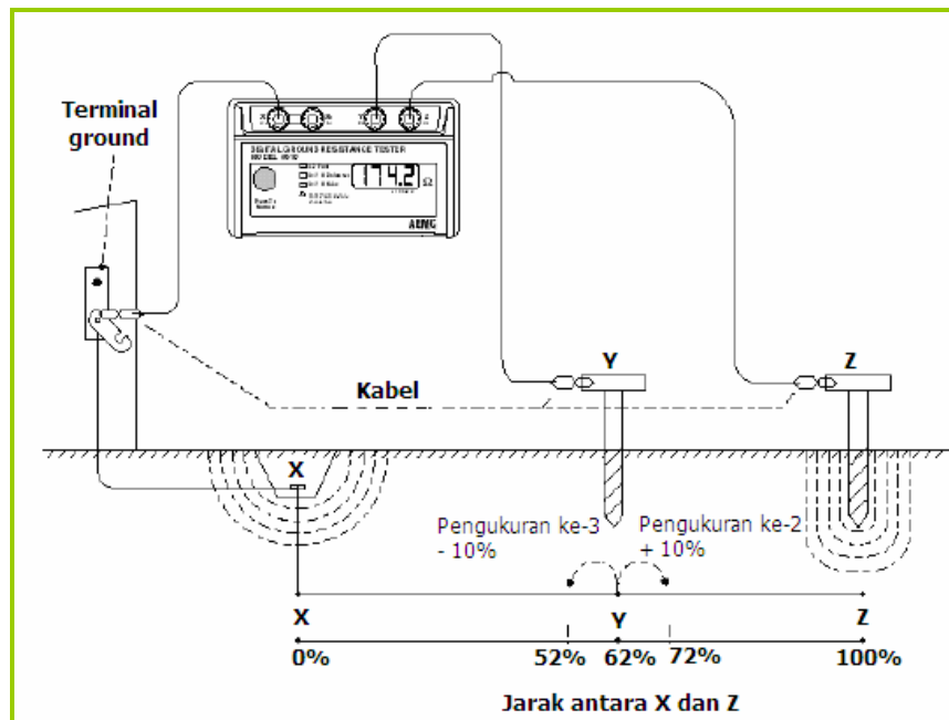
Gambar 2.120 Pengukuran resistansi elektroda pentanahan menggunakan Metoda 62%
