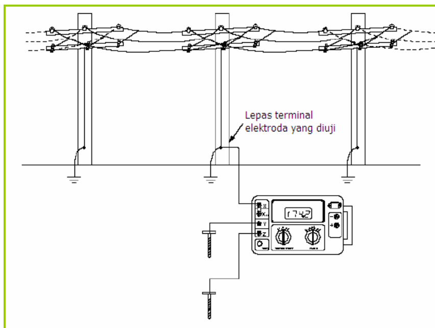
Gambar 2.128 Cara menghindari noise dengan pengaturan rentangan kabel-kabel ukur
