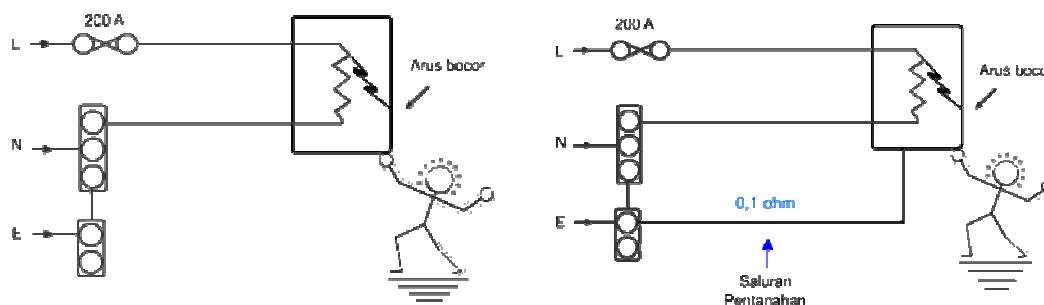
Gambar 2.110 Tegangan sentuh tidak langsung
