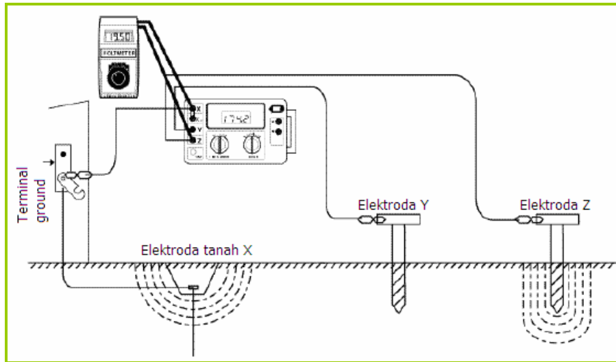
Gambar 2.126 Metoda pengukuran derau dalam sistem pentanahan
