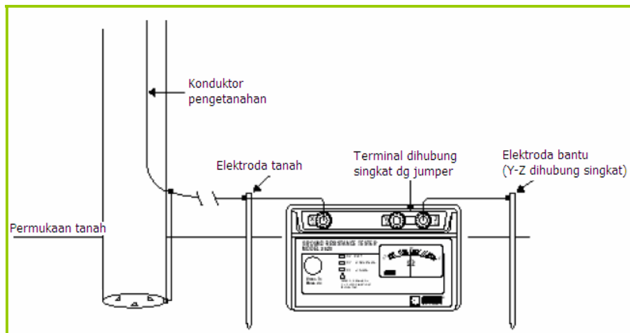
Gambar 2.124 Metoda pengukuran dua-titik
