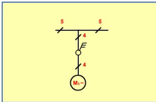
c. Gambar saluran listrik saklar kutub tiga
