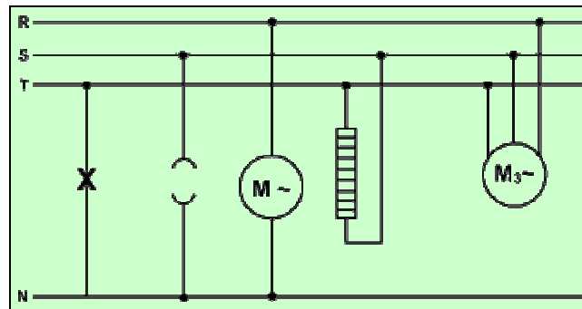
Gambar 2.33 Rangkaian macam-macam Beban Sistem 3 fasa, 4 kawat
