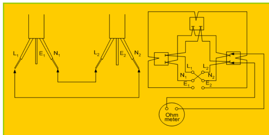
Gambar 2.134 Pengukuran resistansi kawat penghantar melingkar fasa dan netral
