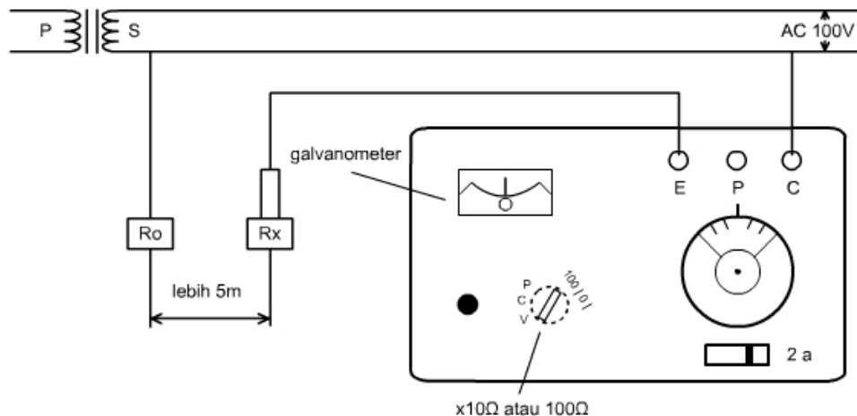
Gambar 2.116 pengukuran Metoda 2 Kutub
