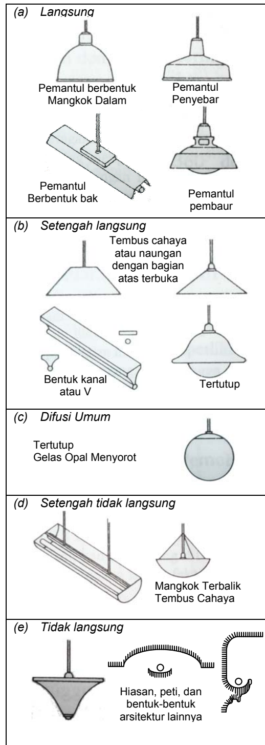
(b) Berbagai bentuk armatur
