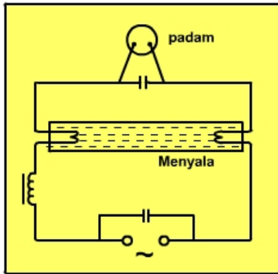
Gambar 2.75 Tahapan Kerja Lampu Fluoresen
