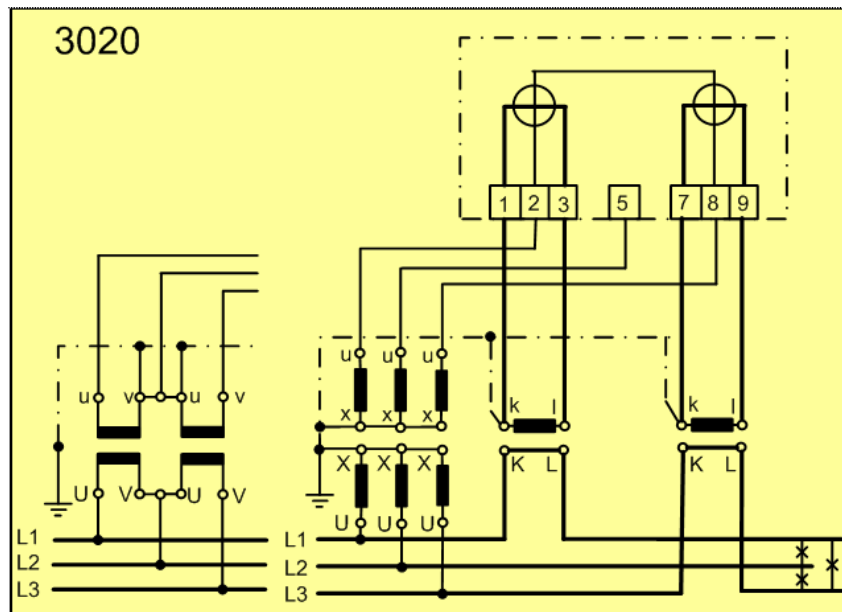
Gambar 2.19 Rangkaian Kwh tiga fasa dengan trafo arus dan trafo tegangan
