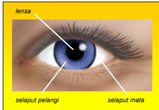
Gambar 2.43 Mata Manusia
