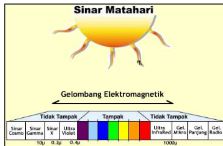
Gambar 2.38 Kelompok Gelombang Elektromagnetik
