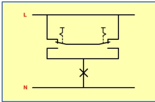
a. Gambar rangkaian listriknya
